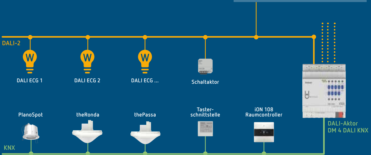
Systemschaubild: Broadcast-Steuerung
